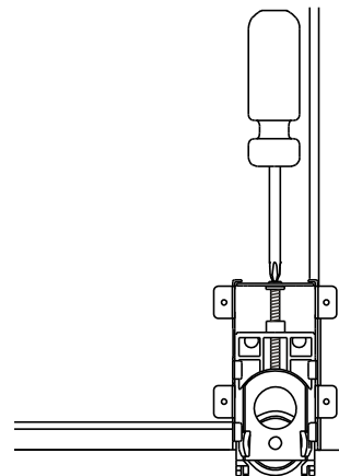
Asennusasento Monteringsställning
