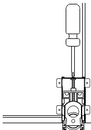
Asennusasento Monteringsställning
